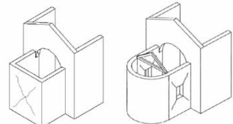
19. ELEMENTI DI COPERTURA: AULA
