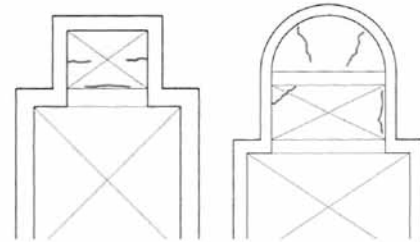
20. ELEMENTI DI COPERTURA: TRANSETTO
