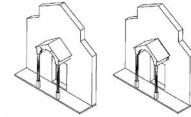
6. MECCANISMI DI TAGLIO NELLE PARETI LATERALI (RISPOSTA LONGITUDINALE)
