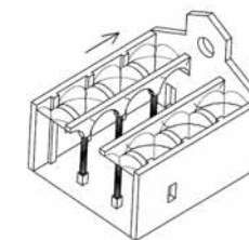
9. VOLTE DELLE NAVATE LATERALI
